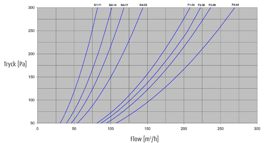
Injusteringsdiagram
