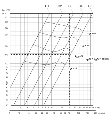
Justeringsdiagram
