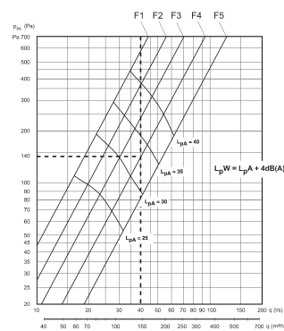
Justeringsdiagram
